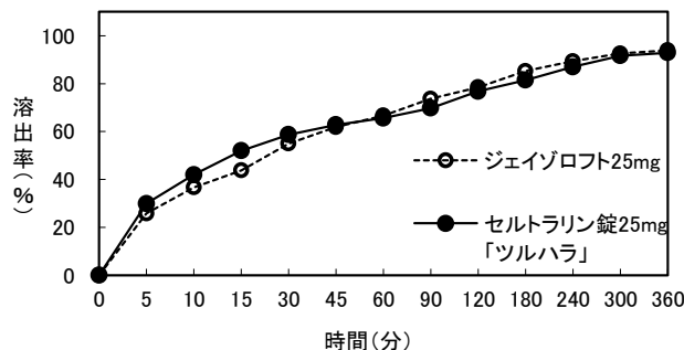
試験液:pH6.8 (回転数:50回転)
