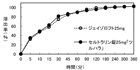
試験液:pH5.0 (回転数:50回転)
